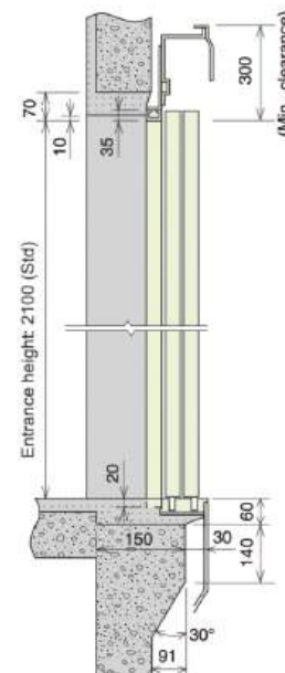
Door elevation (section A-A)
